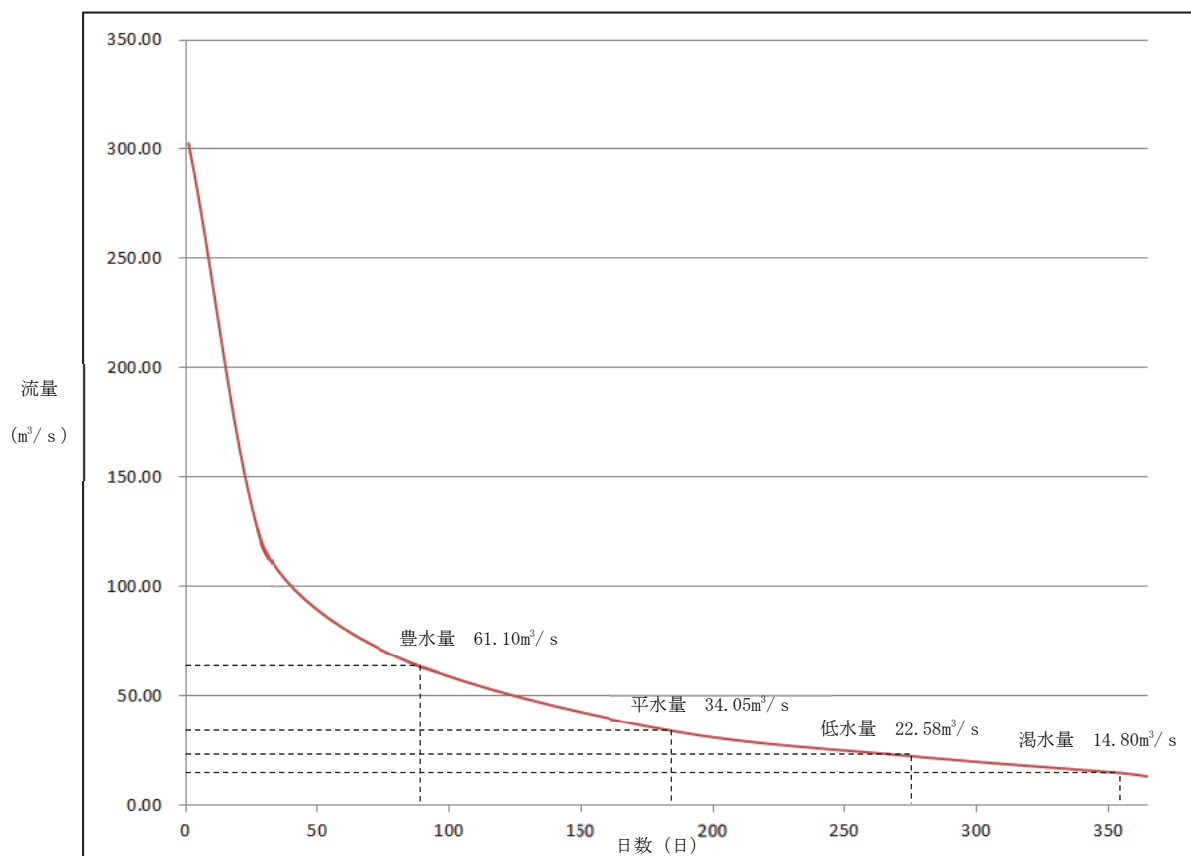
第 1-3-11 図 姫川第六発電所取水堰堤地点流況曲線図
