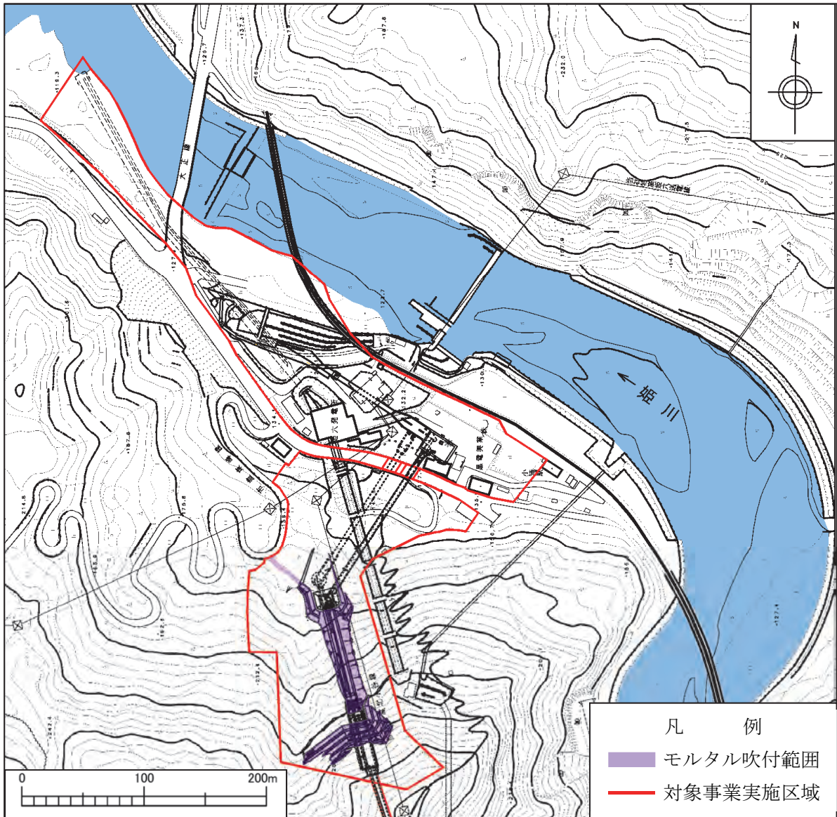
第 1-3-9 図 (2) モルタル吹付範囲 (発電所工事)
