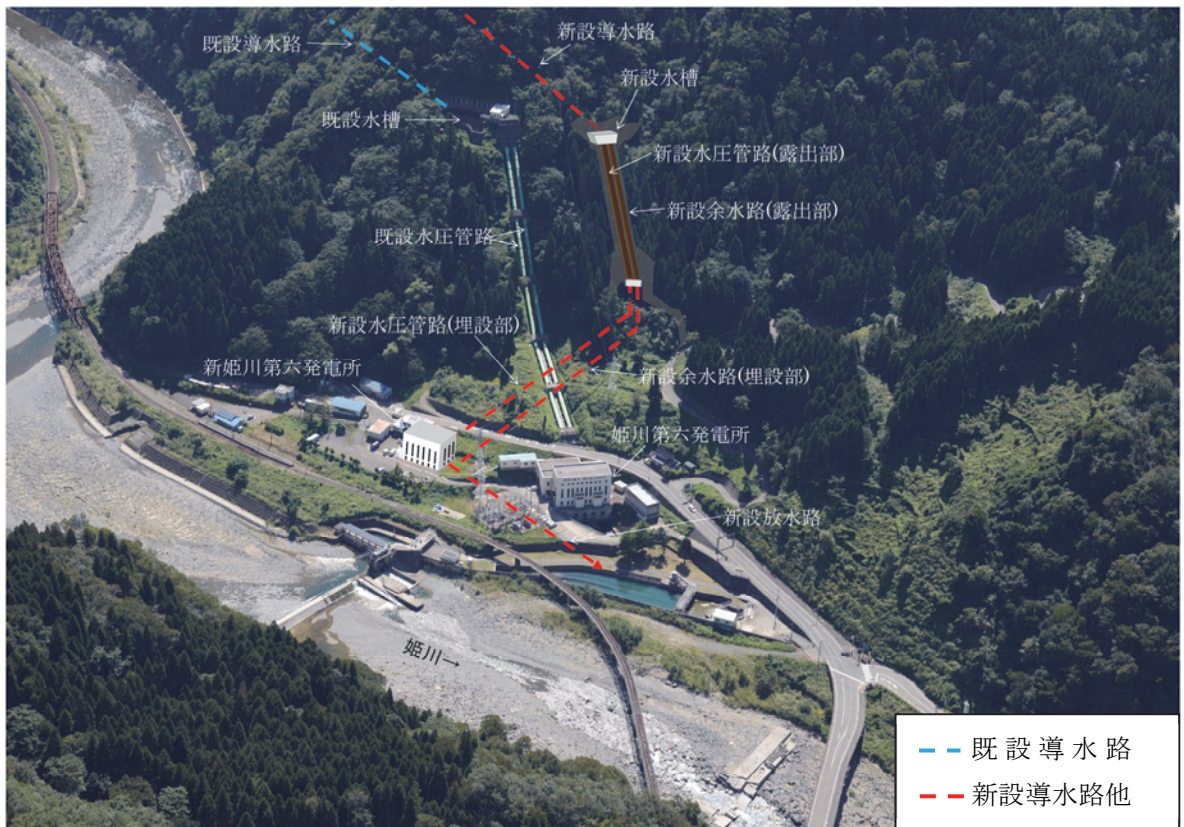
第 1-3-5 図(2) 発電所完成予想図
