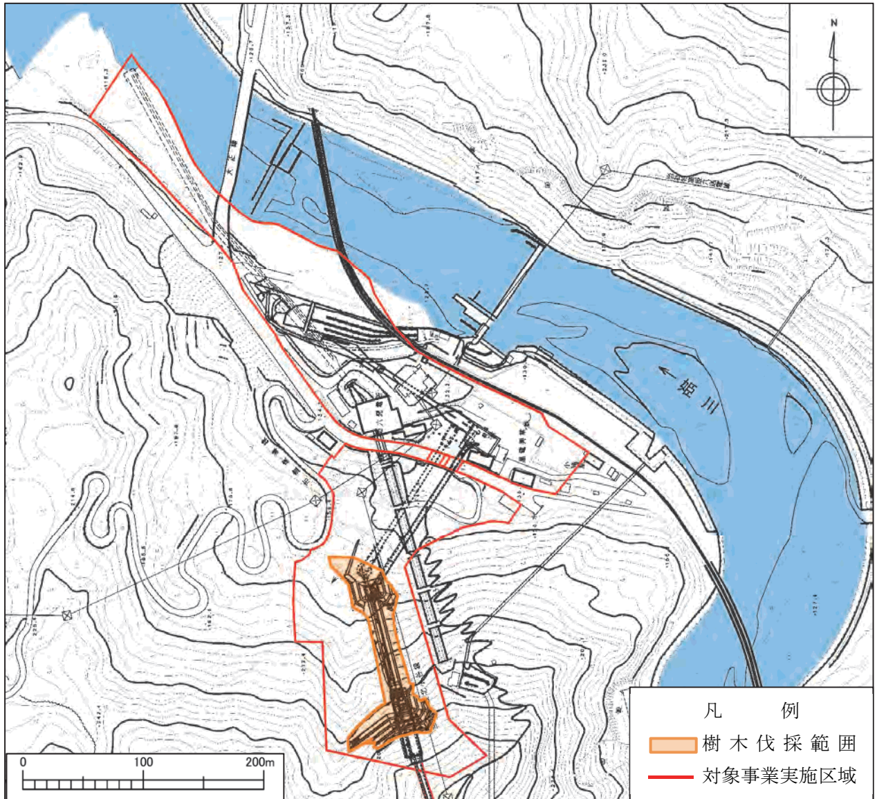
第 1-3-8 図(2) 樹木伐採の範囲 (発電所工事)
