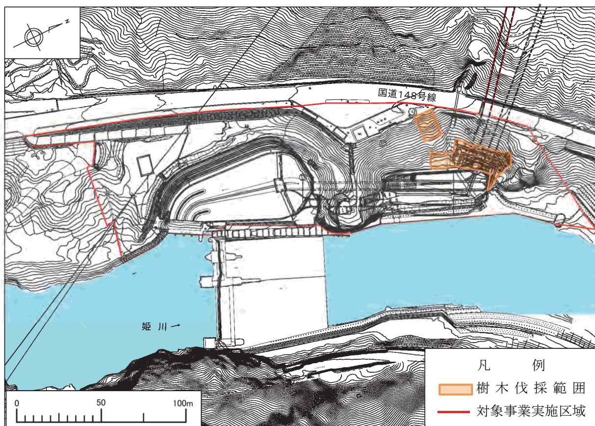
第 1-3-8(1) 図 樹木伐採の範囲 (取水口工事)
