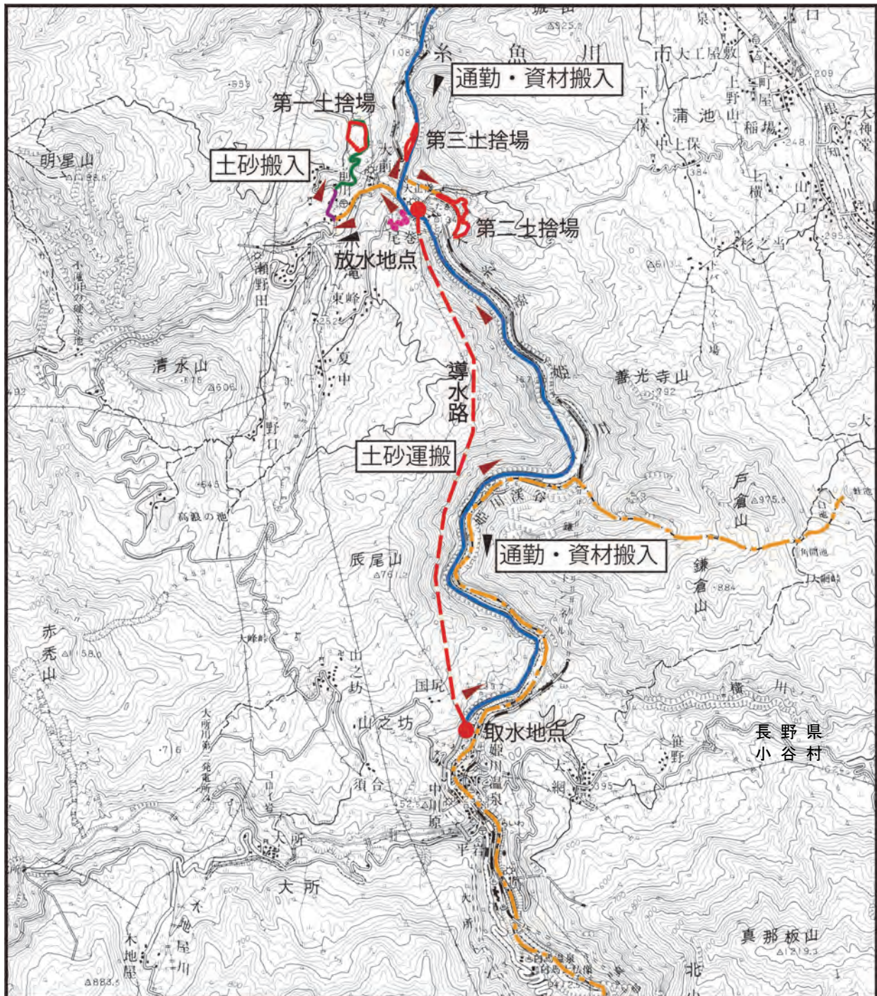
第 1-3-6 図 工所用交通ルートの概要
