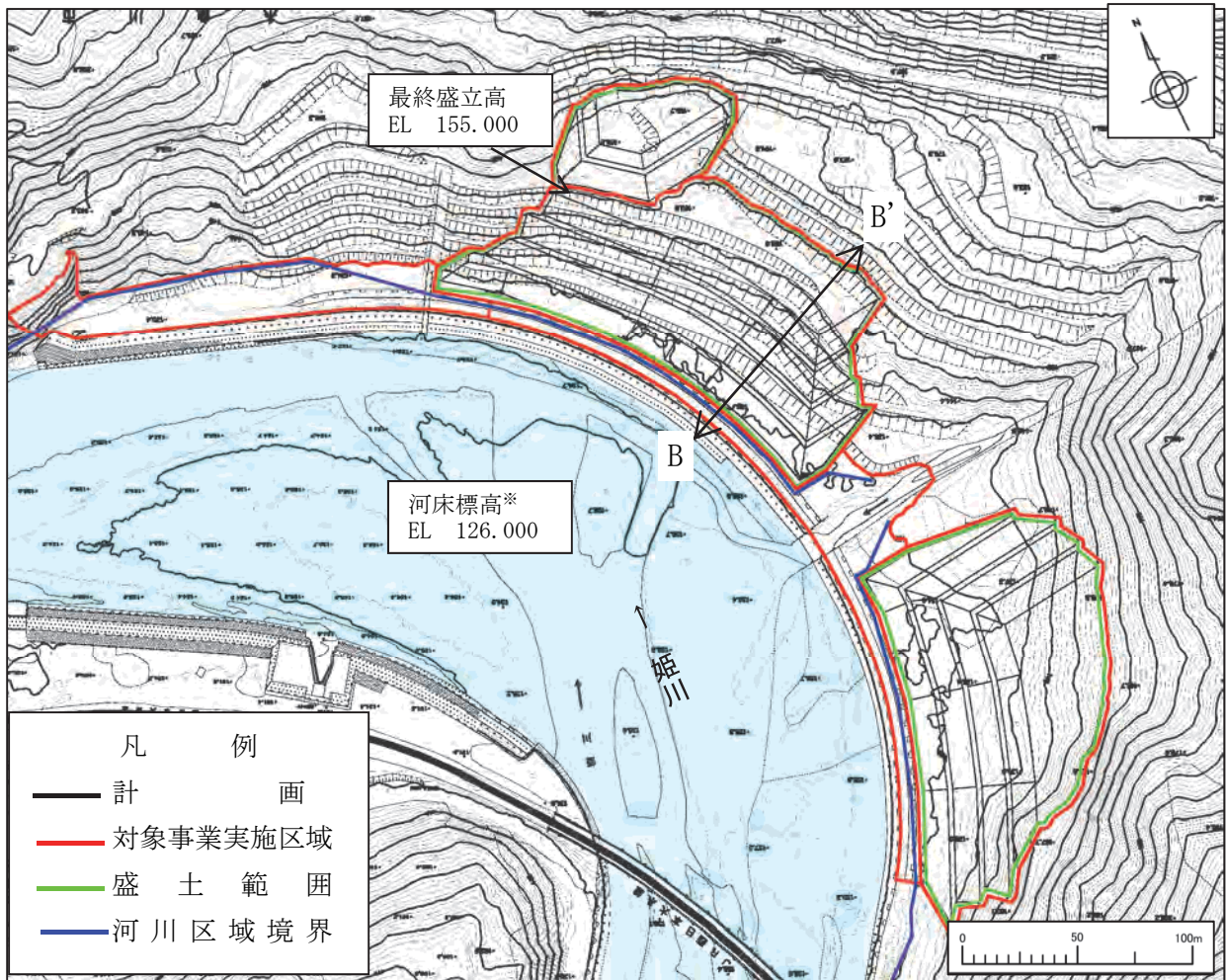
第 1-3-10 図(3) 第二土捨場計画図 (平面図)
