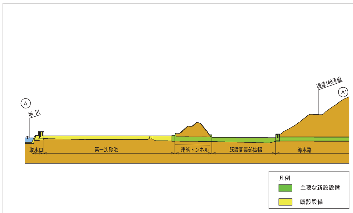
第 1-3-4 図(2) 発電所配置計画の概要（A-A' 断面図）
