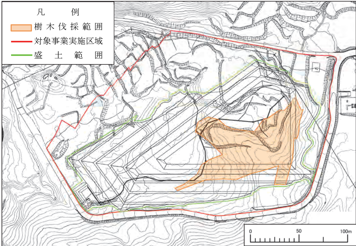
第 1-3-8 図 (3) 樹木伐採の範囲 (第一土捨場)
