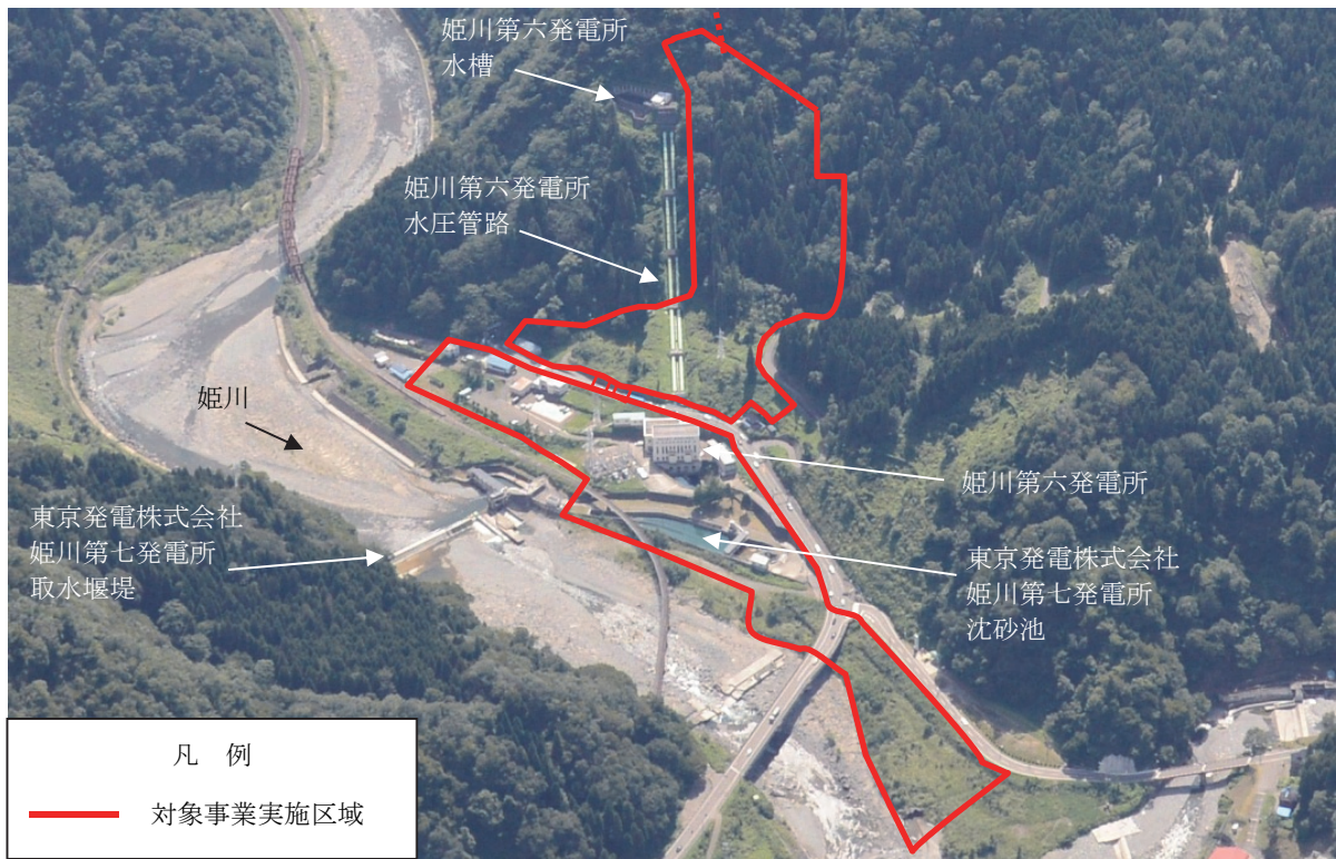
第1-3-3図(2) 対象事業実施区域の鳥瞰図(発電所地点)
