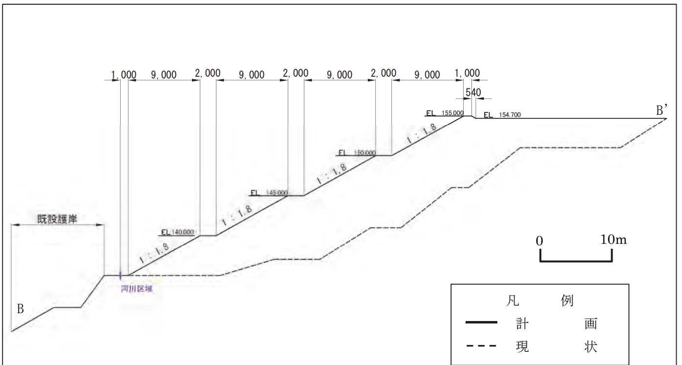
第 1-3-10 図(4) 第二土捨場計画図 (B-B' 断面図)
