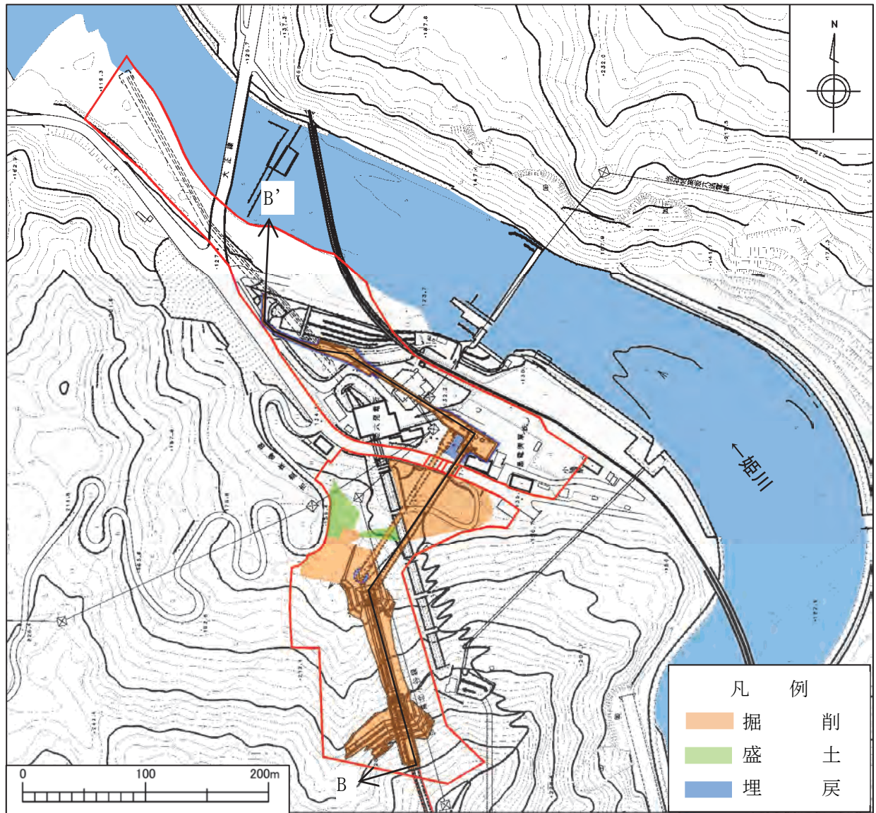
第 1-3-7 図(3) 切取、盛土の工事範囲 (発電所工事、仮設工事)
