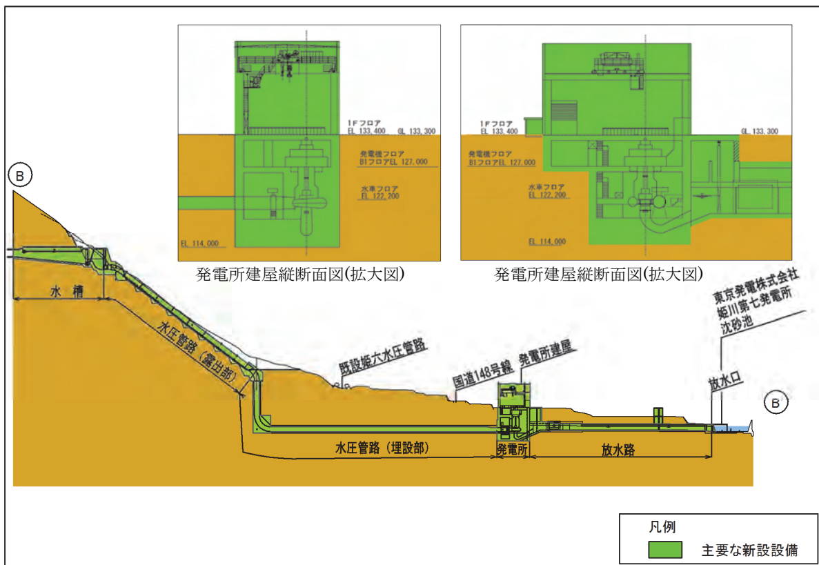
第 1-3-4 図(4) 発電所配置計画の概要 (B-B' 断面図)
