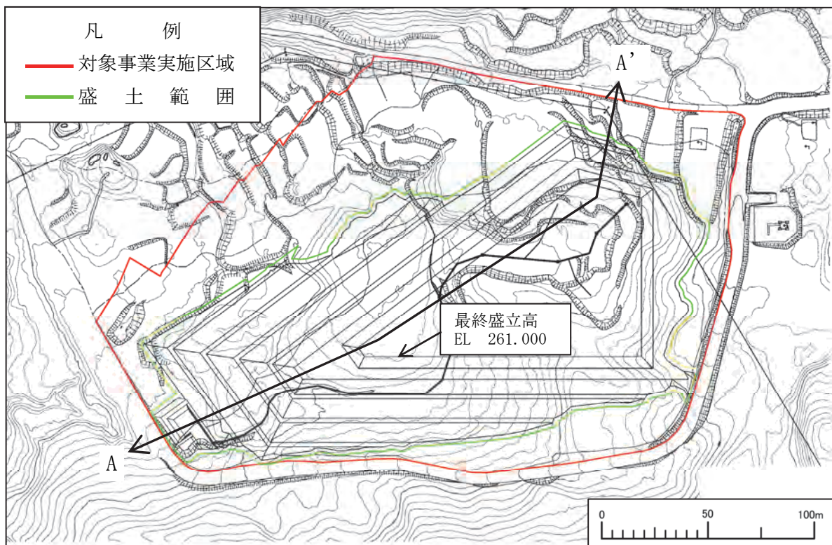
第 1-3-10 図(1) 第一土捨場計画図 (平面図)
