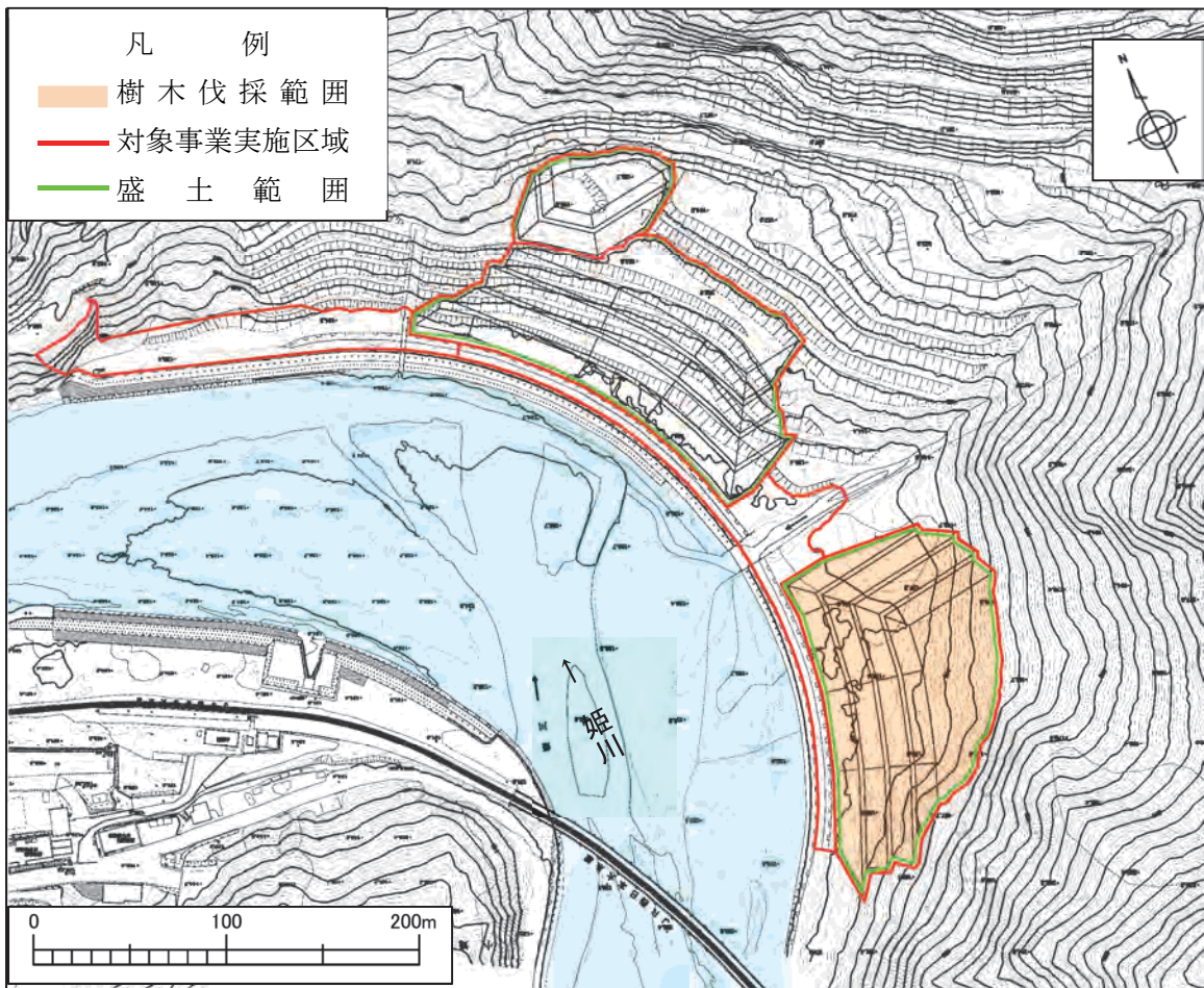
第 1-3-8 図 (4) 樹木伐採の範囲 (第二土捨場)
