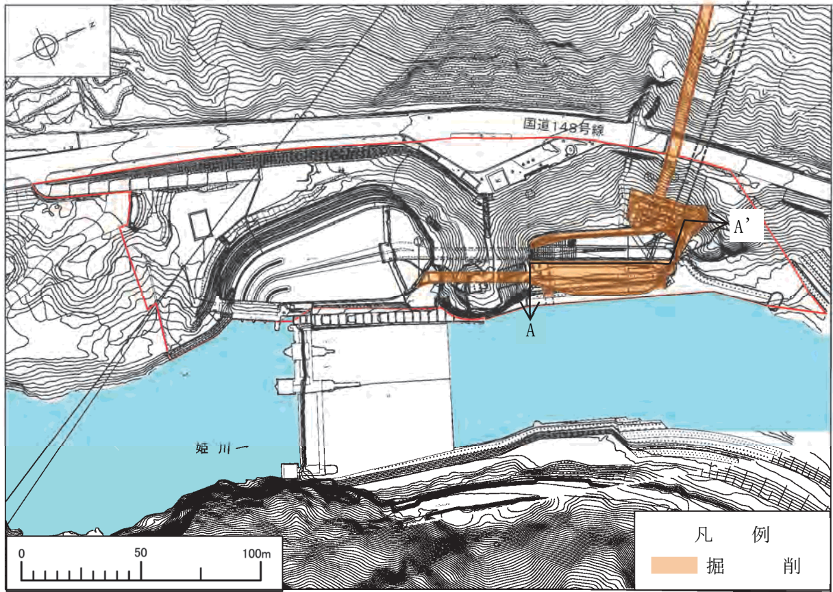
第 1-3-7 図(1) 切取、盛土の工事範囲 (取水口工事)
