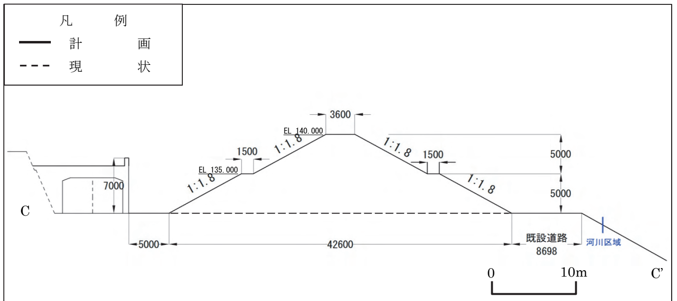
第 1-3-10 図(6) 第三土捨場（土砂仮置場）計画図（C-C' 断面図）
