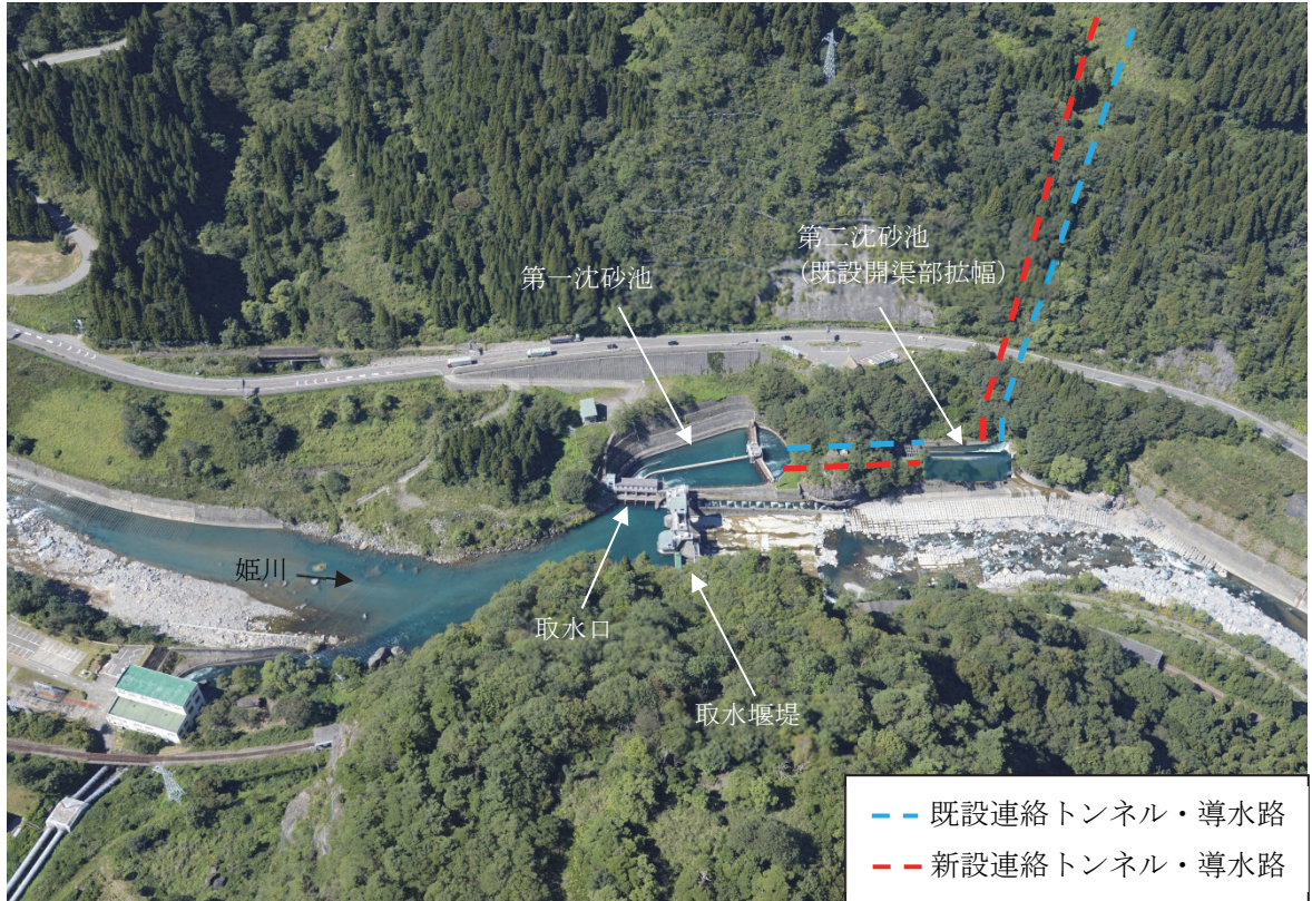
第 1-3-5 図(1) 取水口完成予想図
