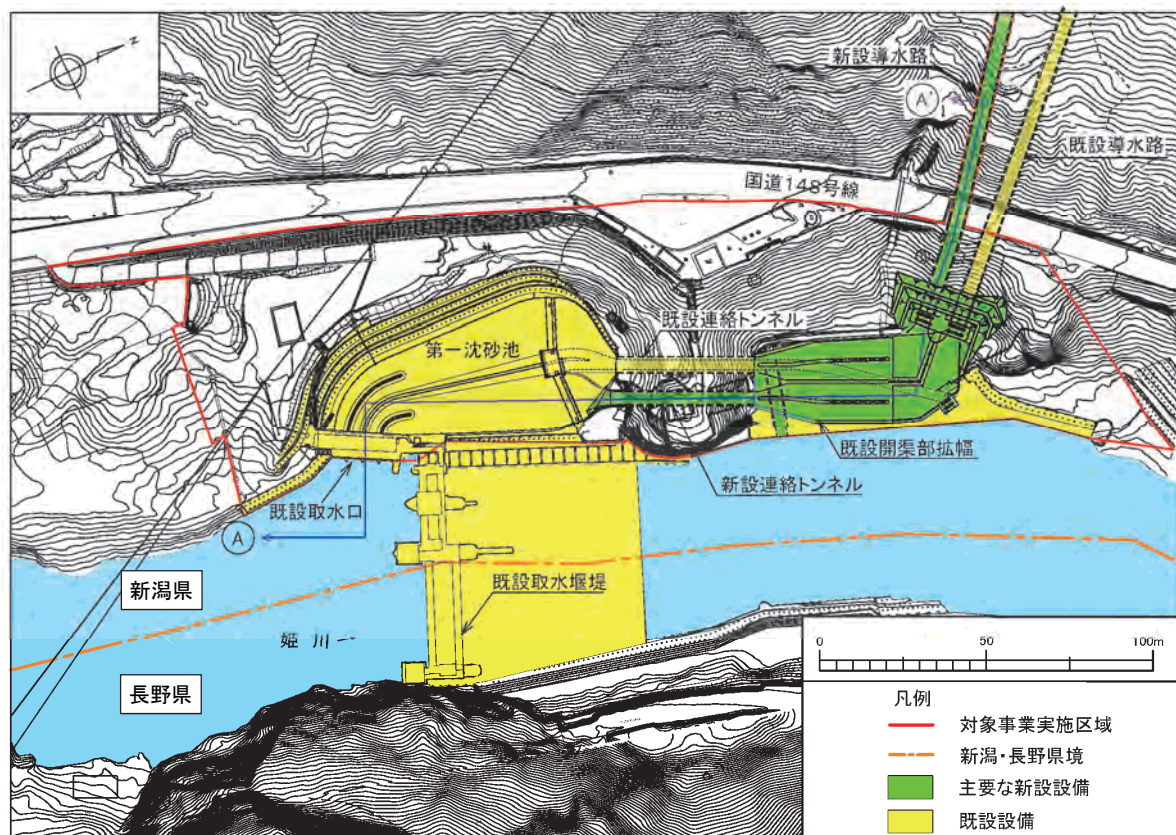
第 1-3-4 図(1) 発電所配置計画の概要（取水口地点平面図）
