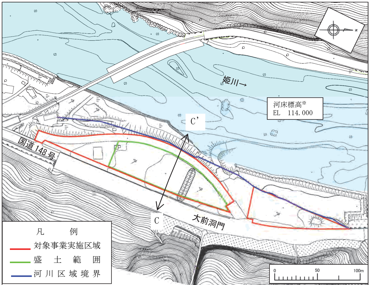
第 1-3-10 図(5) 第三土捨場（土砂仮置場）計画図（平面図）
