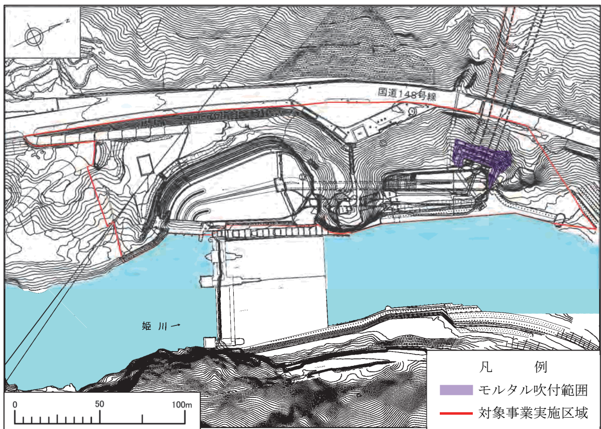
第1-3-9図(1) モルタル吹付範囲(取水口工事)
