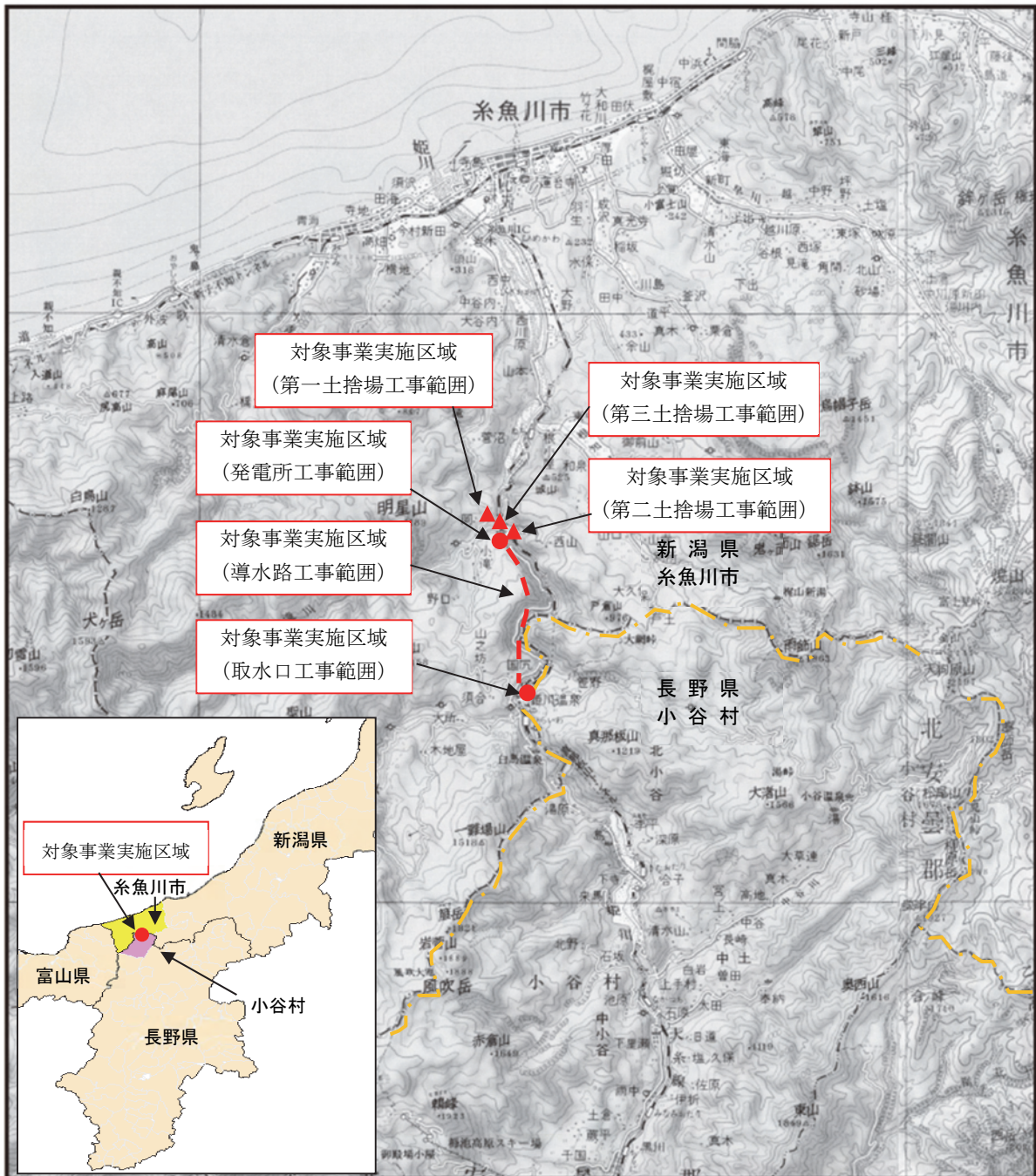
第 1-3-1 図 対象事業実施区域の位置
