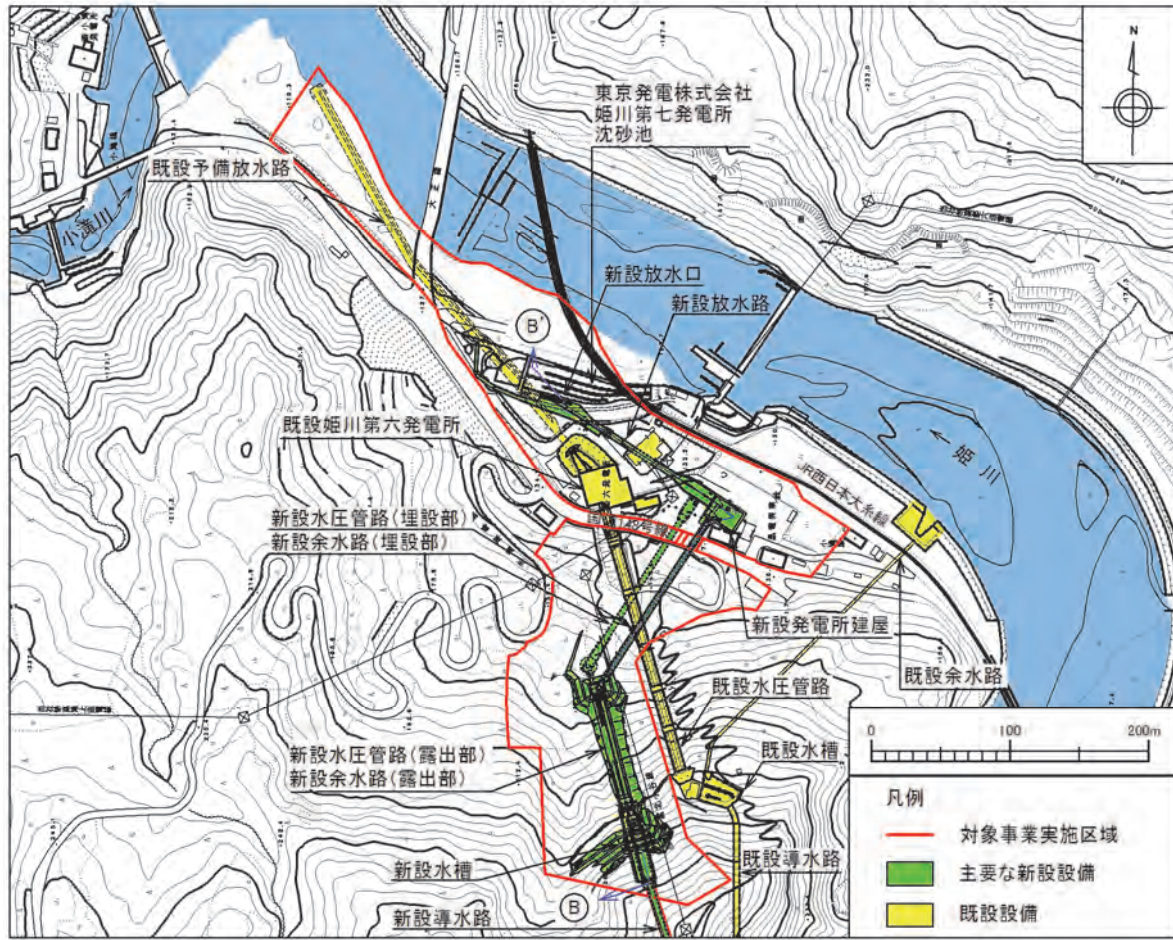
第 1-3-4 図(3) 発電所配置計画の概要 (発電所地点平面図)
