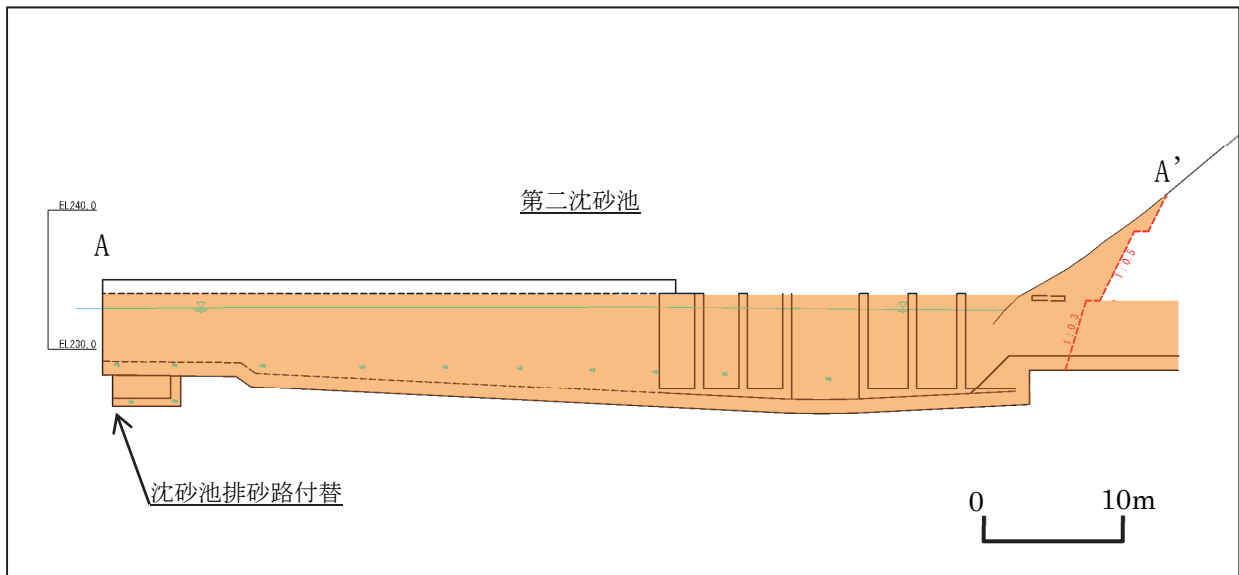
第 1-3-7 図(2) 切取、盛土等の断面 (取水口工事) A-A' 断面図
